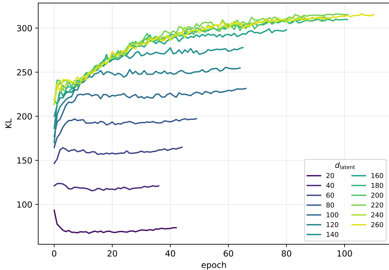
Validation KL
